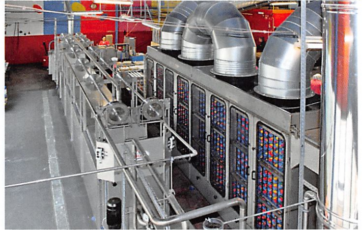
Diese topmoderne Anlage dient in Thannhausen dem Kochen und Färben der Eier. Pro Saison ergibt sich dann die schier unglaubliche Zahl von rund 10 Millionen bunten Eiern.
